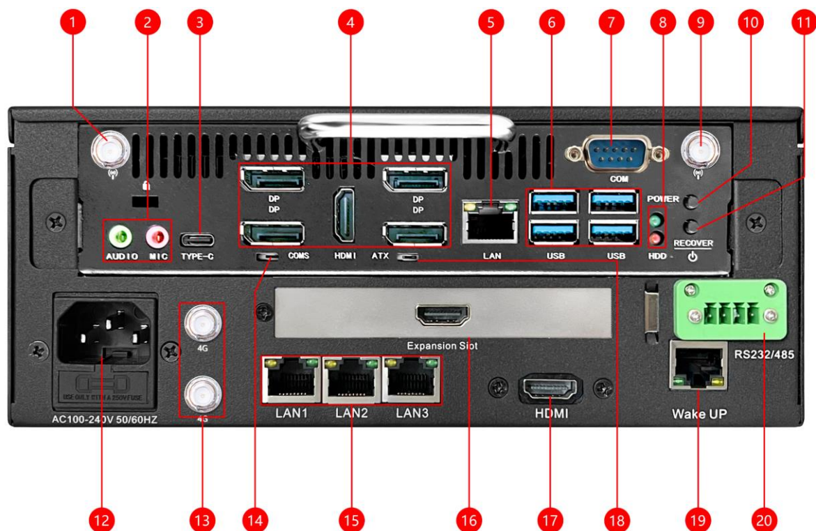
后面板
